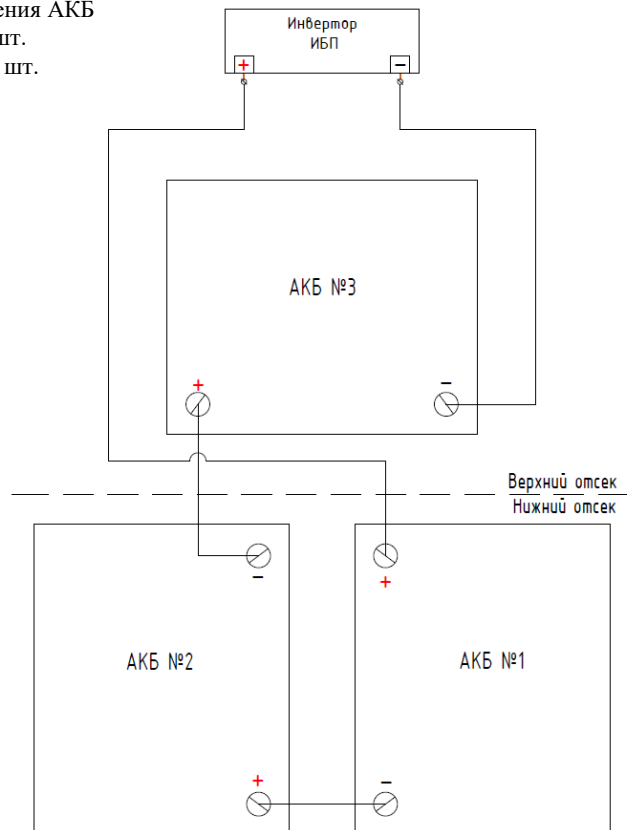
Рис. №2 Схема подключения аккумуляторных батарей.
