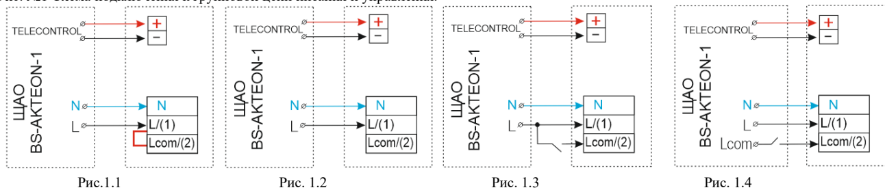
Рис. №1 Схема подключения к групповой цепи питания и управления.
