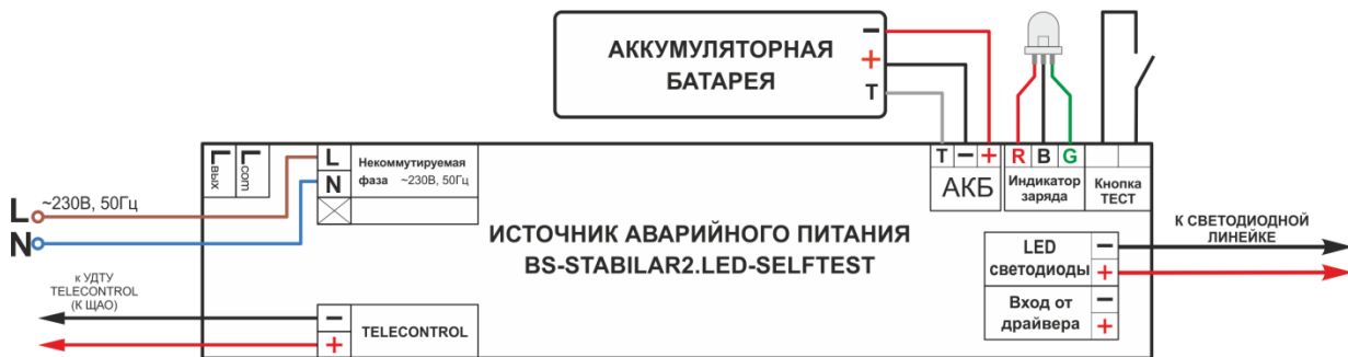
Рис. 2 Схема подключения БАП для аварийного светового прибора в непостоянном режиме:
