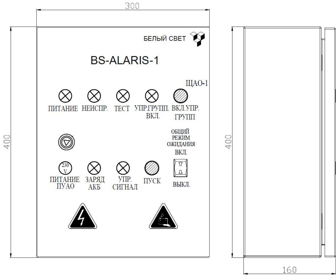
Рис. №2 Установочный чертёж.
