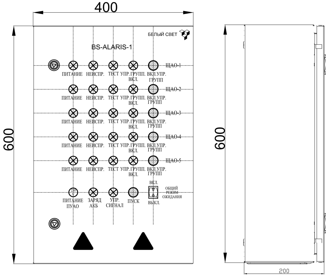
Рис. №2 Установочный чертёж.
