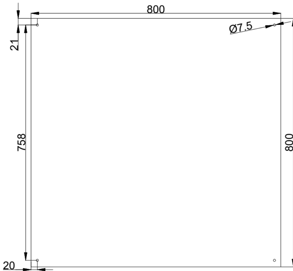
Рис. №2 Установочный чертёж.
