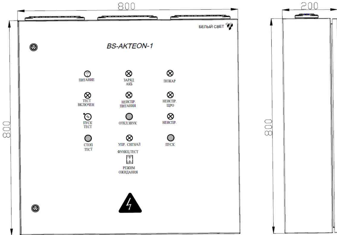
Рис. №2 Установочный чертёж.
