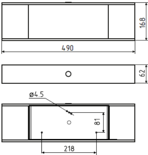
Рис. №2 Габаритный чертёж.
