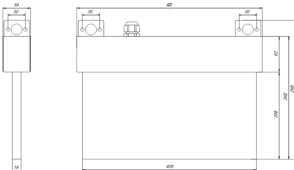
Рис. №2 Габаритный чертёж.
