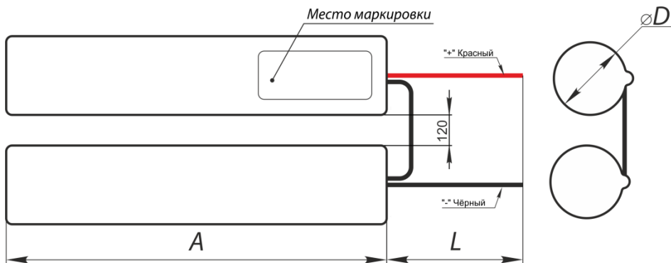
Рис.8 Габаритные размеры Батарея BS-3+3KRHT33/62-4.5/L-NB500-0-1 a18272
