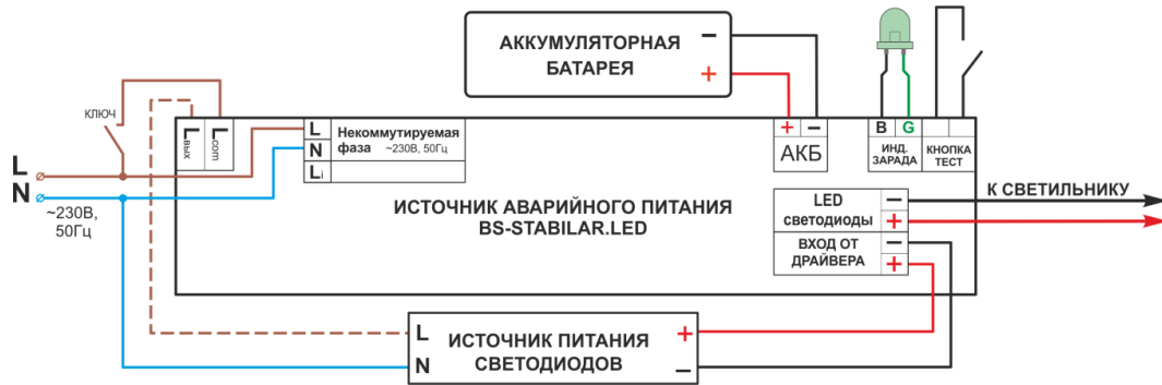
Рис. 2 Схема подключения BS-STABILAR-83-B4-LED OEM-10 для аварийного светового прибора в непостоянном режиме:
