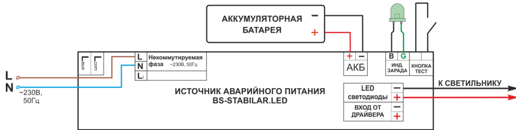
Рис. 2 Схема подключения BS-STABILAR-83-B4-LED OEM-10 для аварийного светового прибора в непостоянном режиме:
