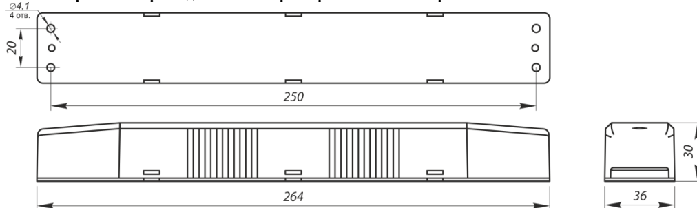
Рис.7 Габаритные и присоединительные размеры источника аварийного питания STABILAR.LED
