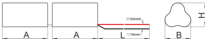
Рис.8 Габаритные размеры BS-3+3KRHT14/50-0,7/A-HB500-0-1
