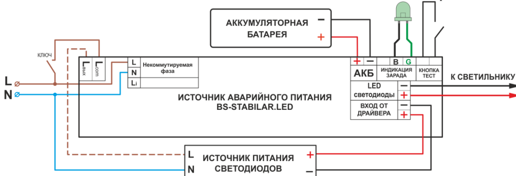
Рис. 1 Схема подключения BS-STABILAR-81-B1-LED и BS-STABILAR-83-B1-LED для аварийного светового прибора в универсальном режиме:
