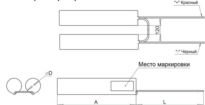
Рис.9 Габаритные размеры BS-3+3KRHT23/43-1.5/L-HB500-0-1 a18268
