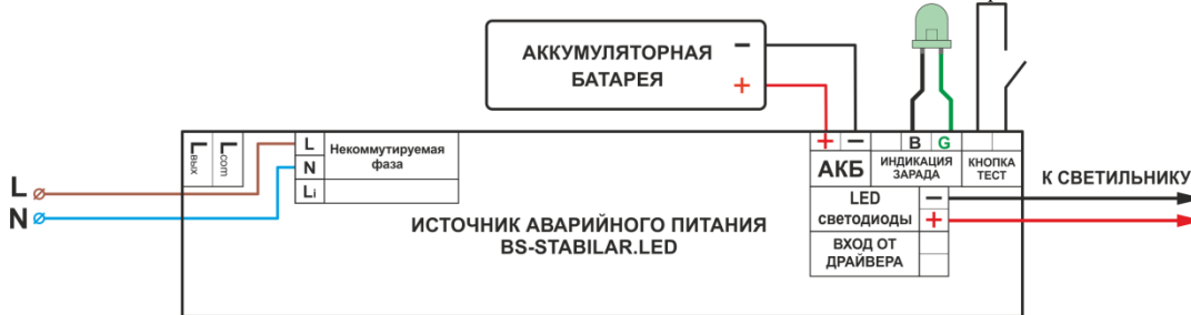
Рис. 2 Схема подключения BS-STABILAR-81-B1-LED и BS-STABILAR-83-B1-LED для аварийного светового прибора в непостоянном режиме:
