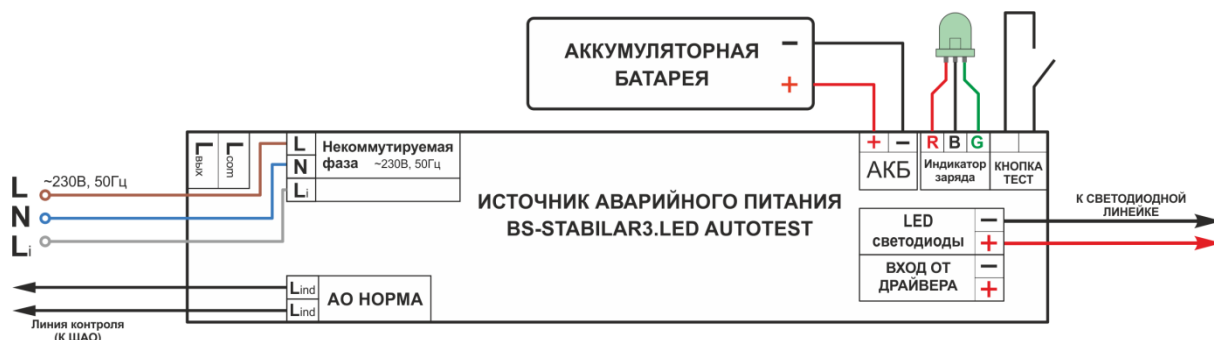
Рис. 2 Схема подключения BS-STABILAR3-81-B2-LED и BS-STABILAR3-83-B2-LED для аварийного светового прибора в непостоянном режиме:
