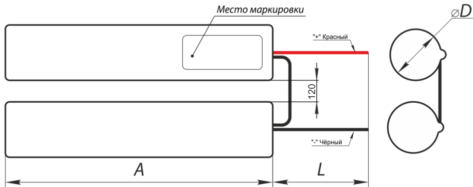
Рис.8 Габаритные размеры батарей
