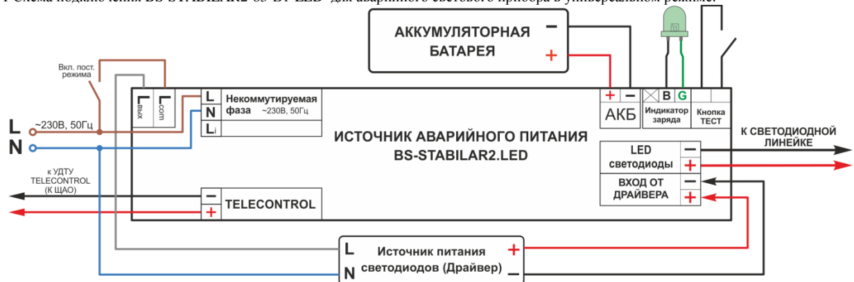
Рис. 1 Схема подключения BS-STABILAR2-83-B1-LED для аварийного светового прибора в универсальном режиме:
