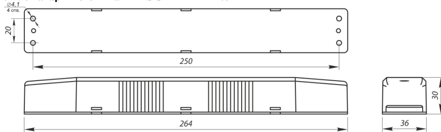
Рис. 9 Блок аварийного питания BS-STABILAR2-83-B1-LED BOX IP30
