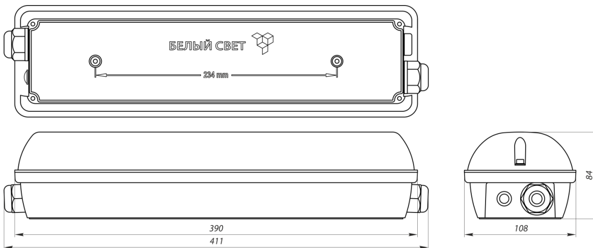
Рис. 10 Блок аварийного питания BS-STABILAR2-83-B1-LED BOX IP66
