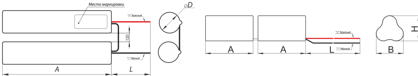
Рис. 7 Батарея BS-3+3KRHT23/43-1.5/L-HB500-0-1 а18268
