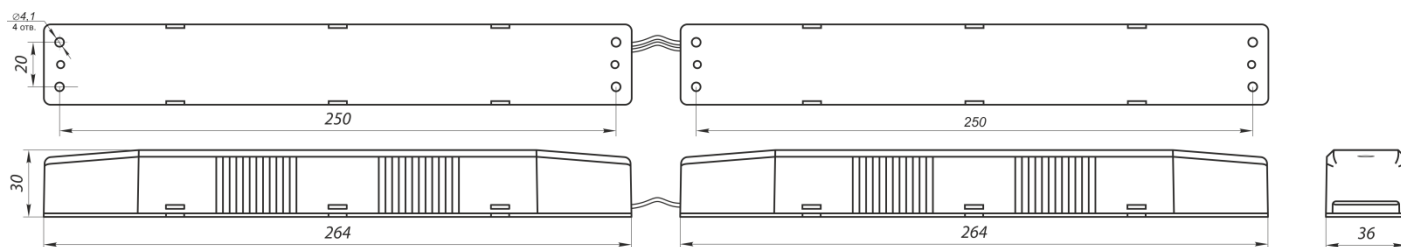
Рис. 10 Блок аварийного питания BS-STABILAR2-83-B1-LED BOX IP66
