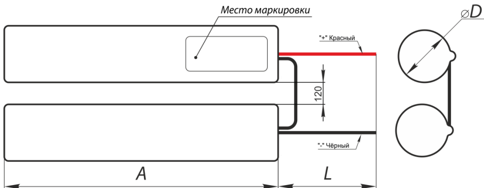
Рис.8 Габаритные размеры Батарея BS-3+3KRHT14/50-0.7/A-НВ500-0-1 а27148
