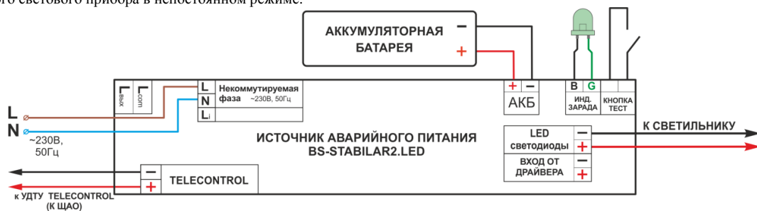
Рис. 2 Схема подключения BS-STABILAR2-81-B3-LED (2,5-200 W / = 50-250 V) OEM-10 для аварийного светового прибора в непостоянном режиме:
