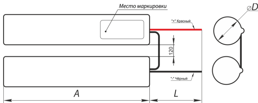
Рис.7 Габаритные размеры Батарея BS-3+3KRHT23/43-1.5/L-НВ500-0-1 и BS-3+3HRHT26/50-4,0/L-НВ500-0-1
