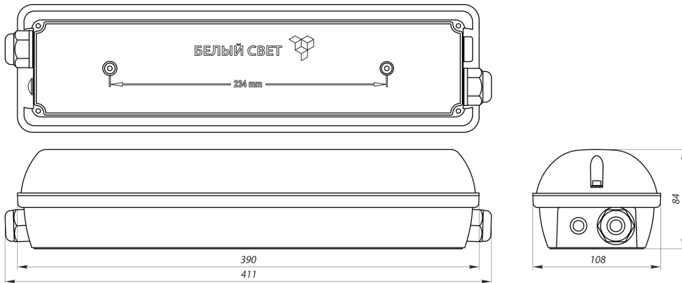
Рис. 8 Блок аварийного питания BS-STABILAR2-81-B4-LED BOX IP66 (6,0-300 W / = 50-250 V) Блок аварийного питания BS-STABILAR2-83-B4-LED BOX IP66 (6,0-300 W / = 50-250 V)
