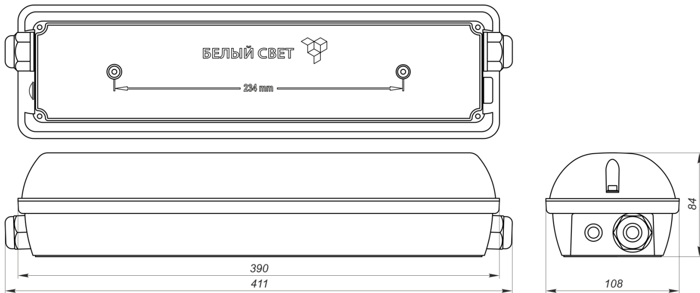
Рис. 6 Блок аварийного питания
