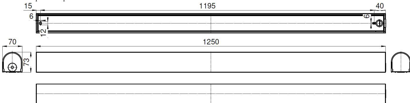
Рис. №2 Габаритный чертёж
