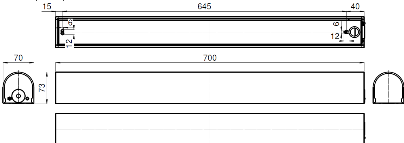
Рис. №5 Габаритный чертёж
