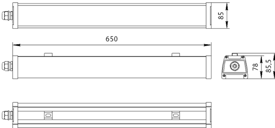
Рис. №5 Габаритный чертёж.
